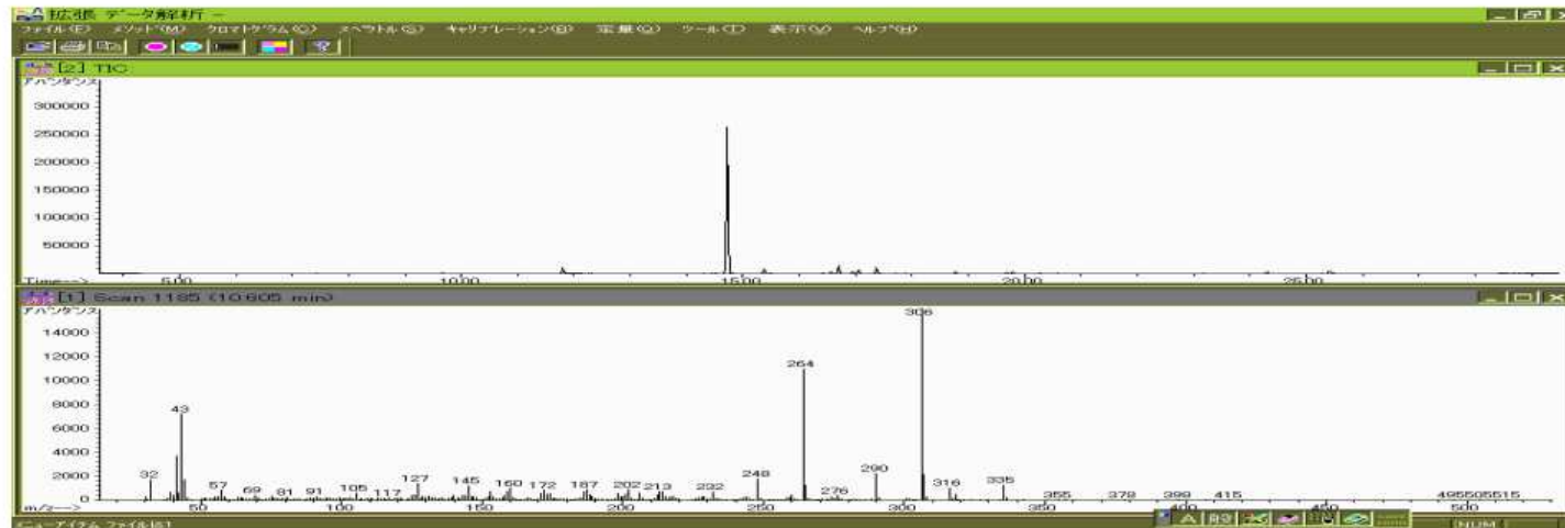
図 1：生姜抽出エキス通常精製（SIM のトータルイオンクロマト；TIC）
