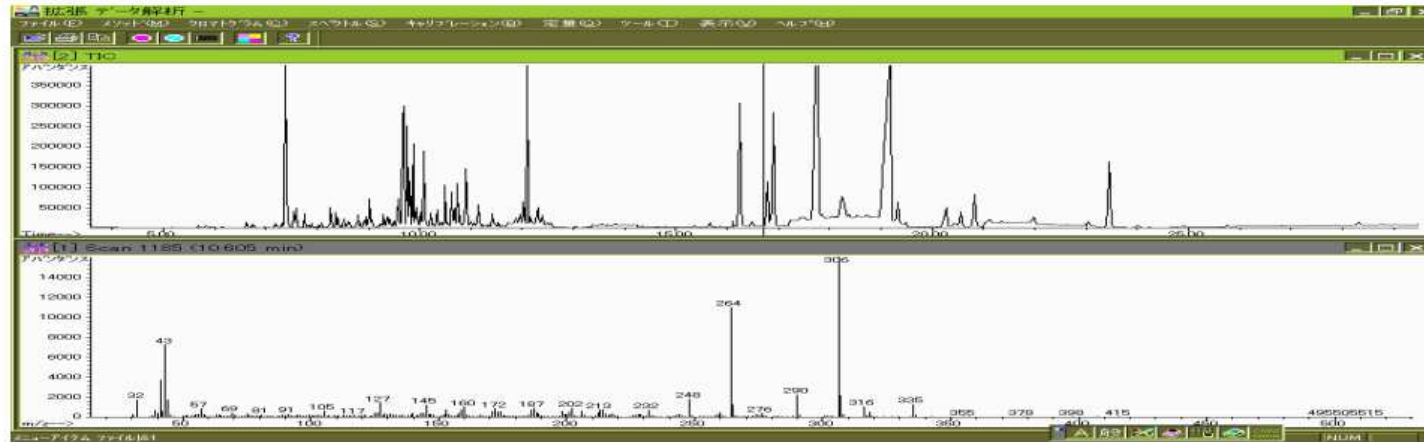
図 1：生姜抽出エキス通常精製（SIM のトータルイオンクロマト；TIC）
